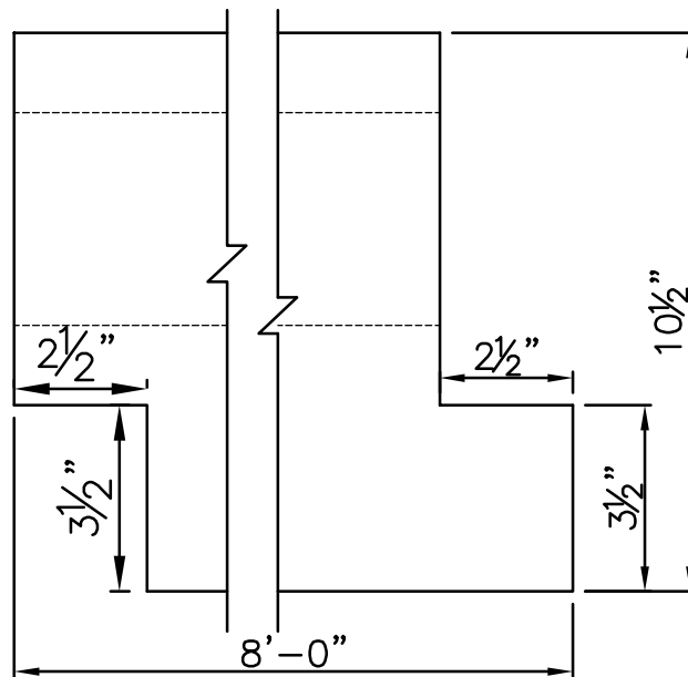
SIDE VEIW
